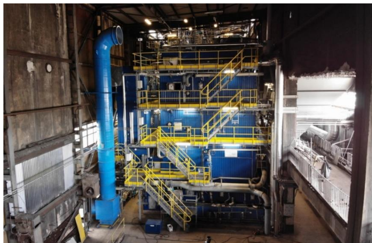
Budowa instalacji ograniczającej emisję zanieczyszczeń do powietrza, Polkowice
